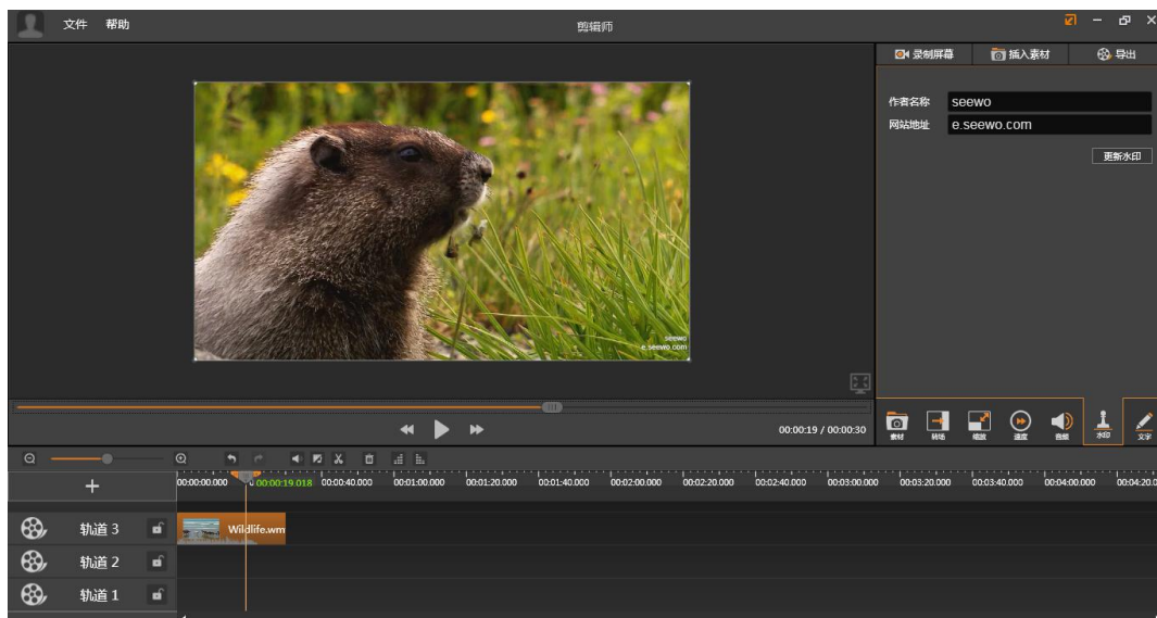
图 3-3-2-4-2 插入水印
