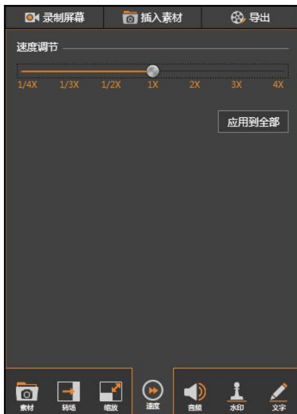
图 3-3-3-5-1 编辑速度
