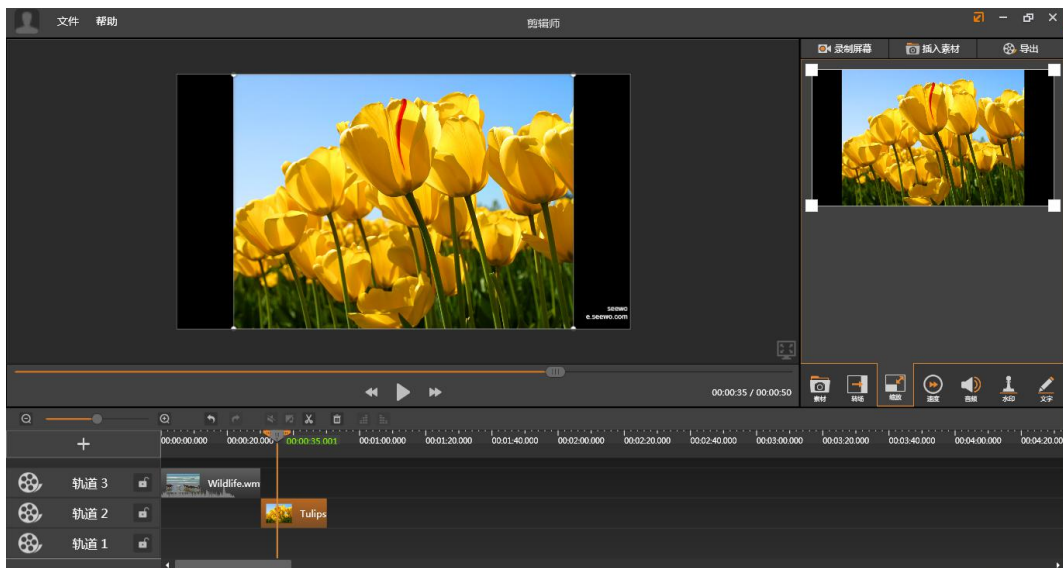
图 3-3-3-1 缩放素材
