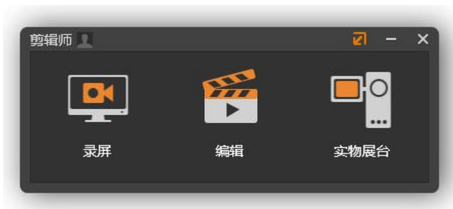
图 3-1-3 主界面
