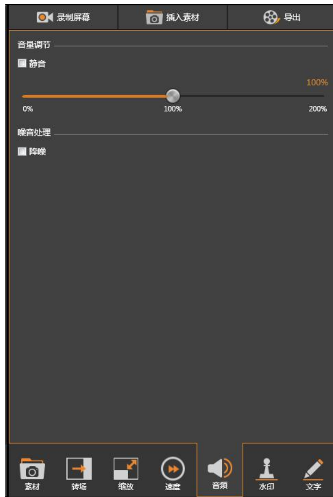
图 3-3-3-6-1 编辑音频
