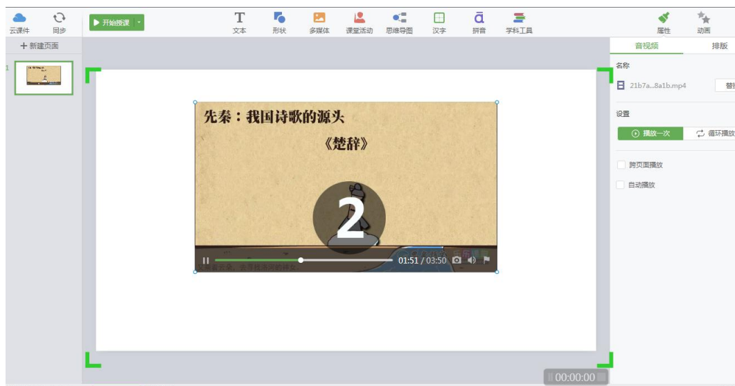
图 3-2-2 录制界面
