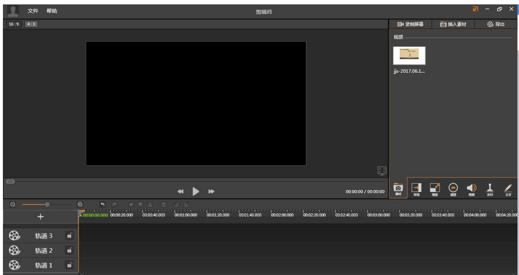
图 3-3 编辑界面
