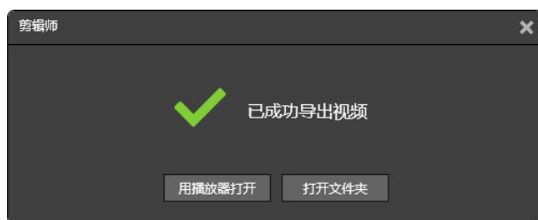
图 3-3-4-3 导出成功
