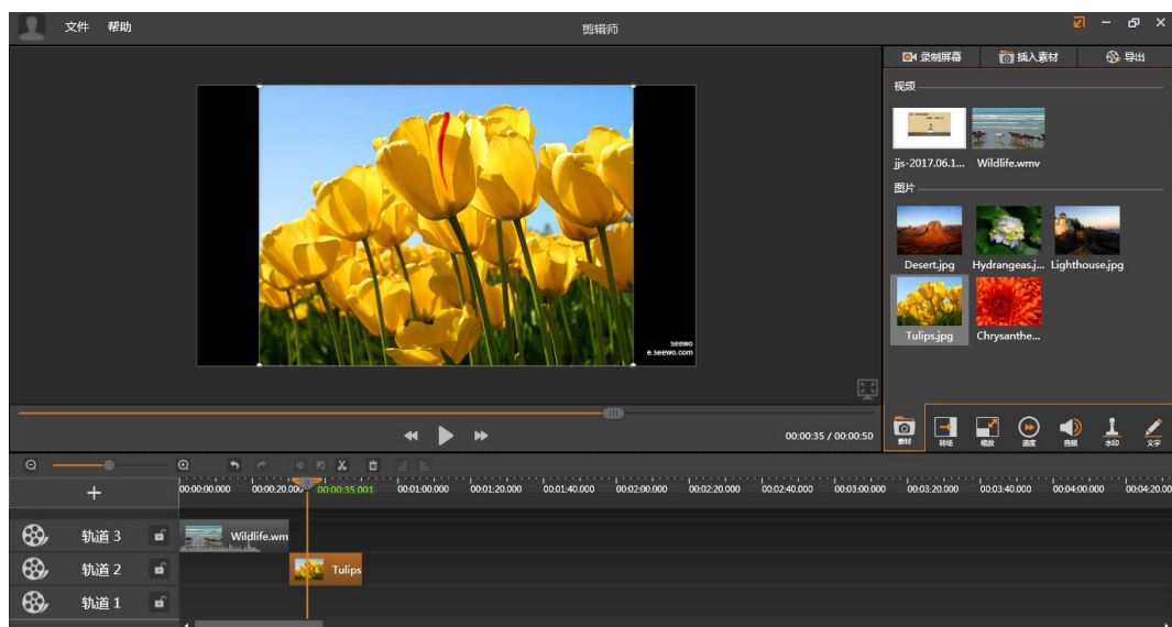
图 3-3-3 素材编辑
